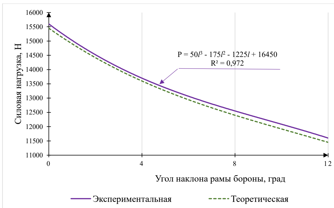
Рисунок 4.10 – Изменение силовой нагрузки, приходящейся на передние движители трактора в зависимости от угла наклона рамы бороны
