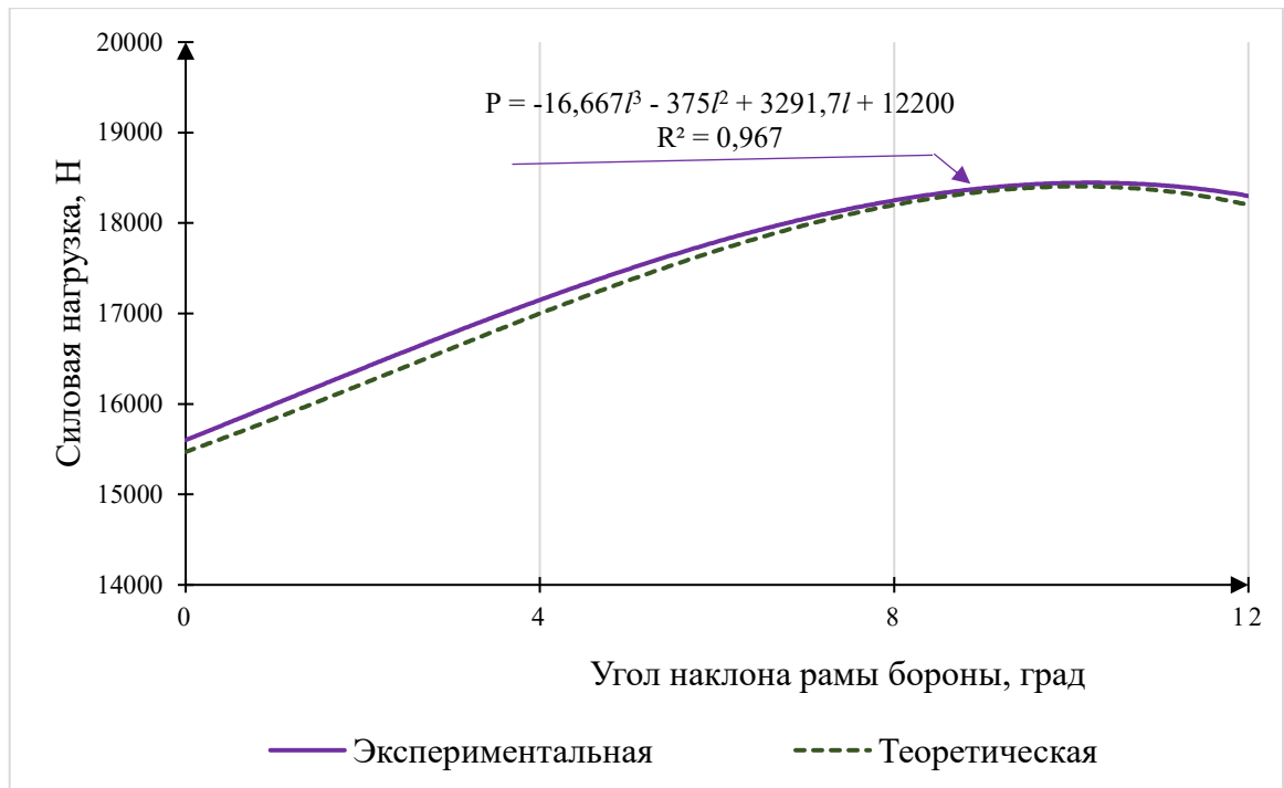
Рисунок 4.14 – Изменение силовой нагрузки, приходящейся на передние движители трактора в зависимости от угла наклона рамы
