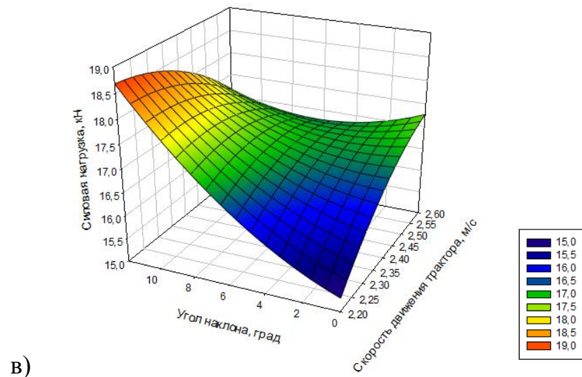
Рисунок 4.32 – Графическая интерпретация зависимости силового воздействия на передние колеса трактора «Беларус-82.1»
