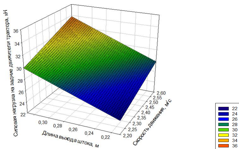
Рисунок 4.24 – Влияние скорости движения и рабочего хода штока гидроцилиндра на тяговое усилие задних движителей трактора при глубине обработки почвы h=18 см
