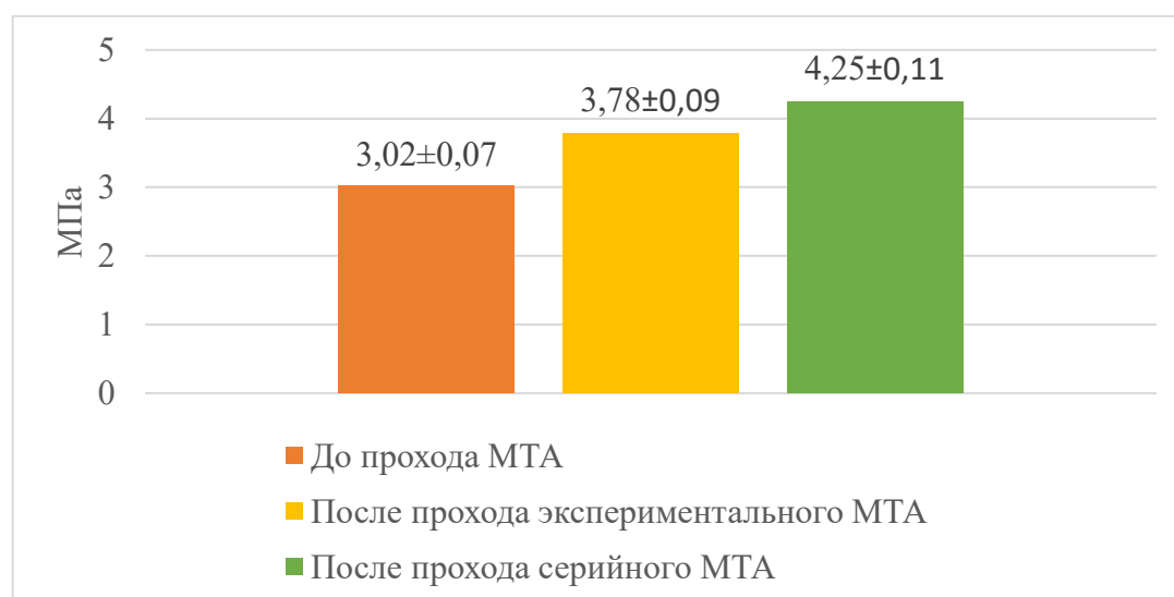
Рисунок 4.17 - Результаты экспериментальных исследований по определению твёрдости почвы по следу трактора
