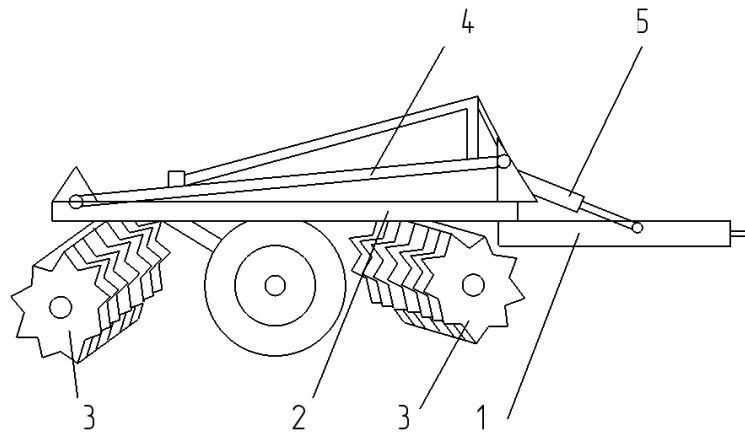
Рисунок 3.5 - Профильный вид МТА с установленным корректором-распределителем силовой нагрузки тяжёлой дисковой бороны
