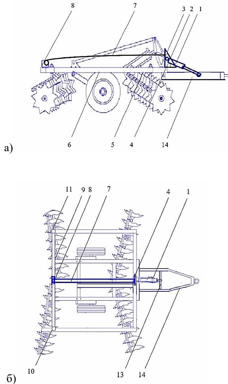
Рисунок 2.3 – Догрузочно-распределяющее устройство для прицепной рамной дисковой бороны (патент РФ на изобретение № 2812473)
