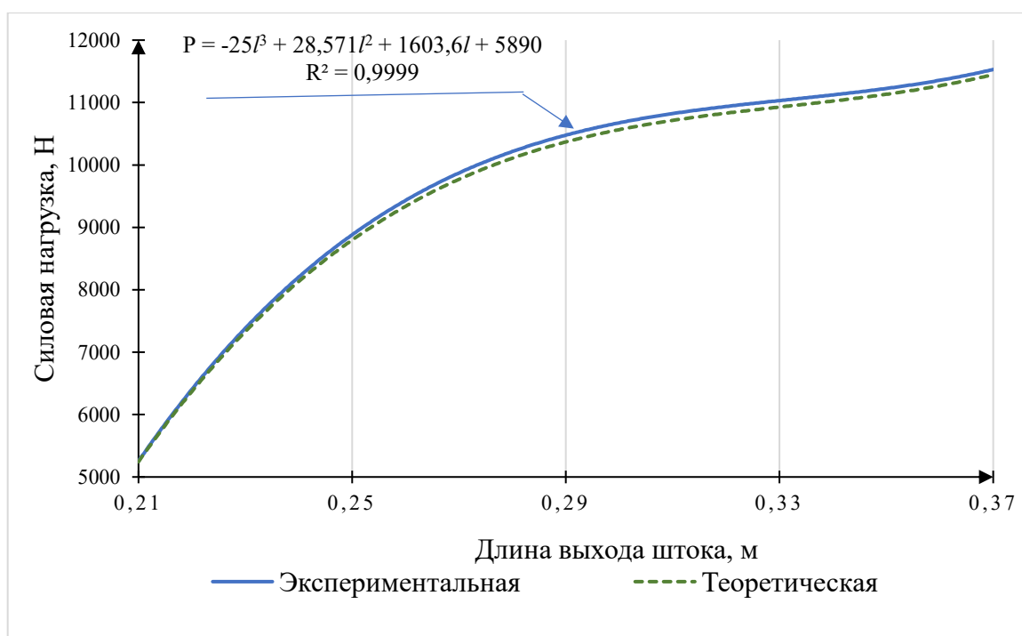
Рисунок 4.3 – Изменение силовой нагрузки, приходящейся на рабочие органы задней секции борона в зависимости от длины выхода штока гидроцилиндра
