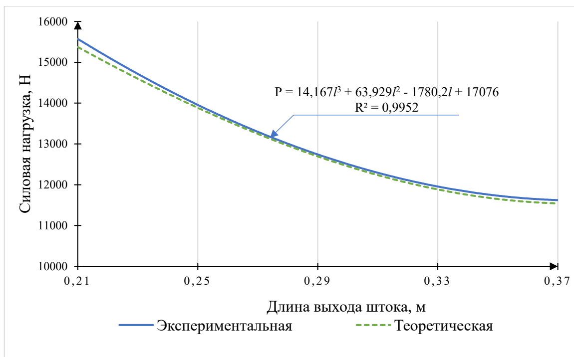
Рисунок 4.2 – Изменение силовой нагрузки, приходящейся на передние движители трактора в зависимости от длины выхода штока гидроцилиндра
