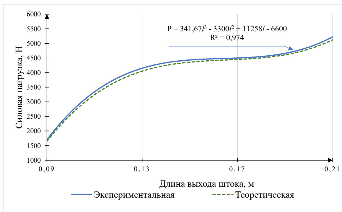
Рисунок 4.7 – Изменение силовой нагрузки, приходящейся на рабочие органы задней секции бороны в зависимости от длины выхода штока гидроцилиндра
