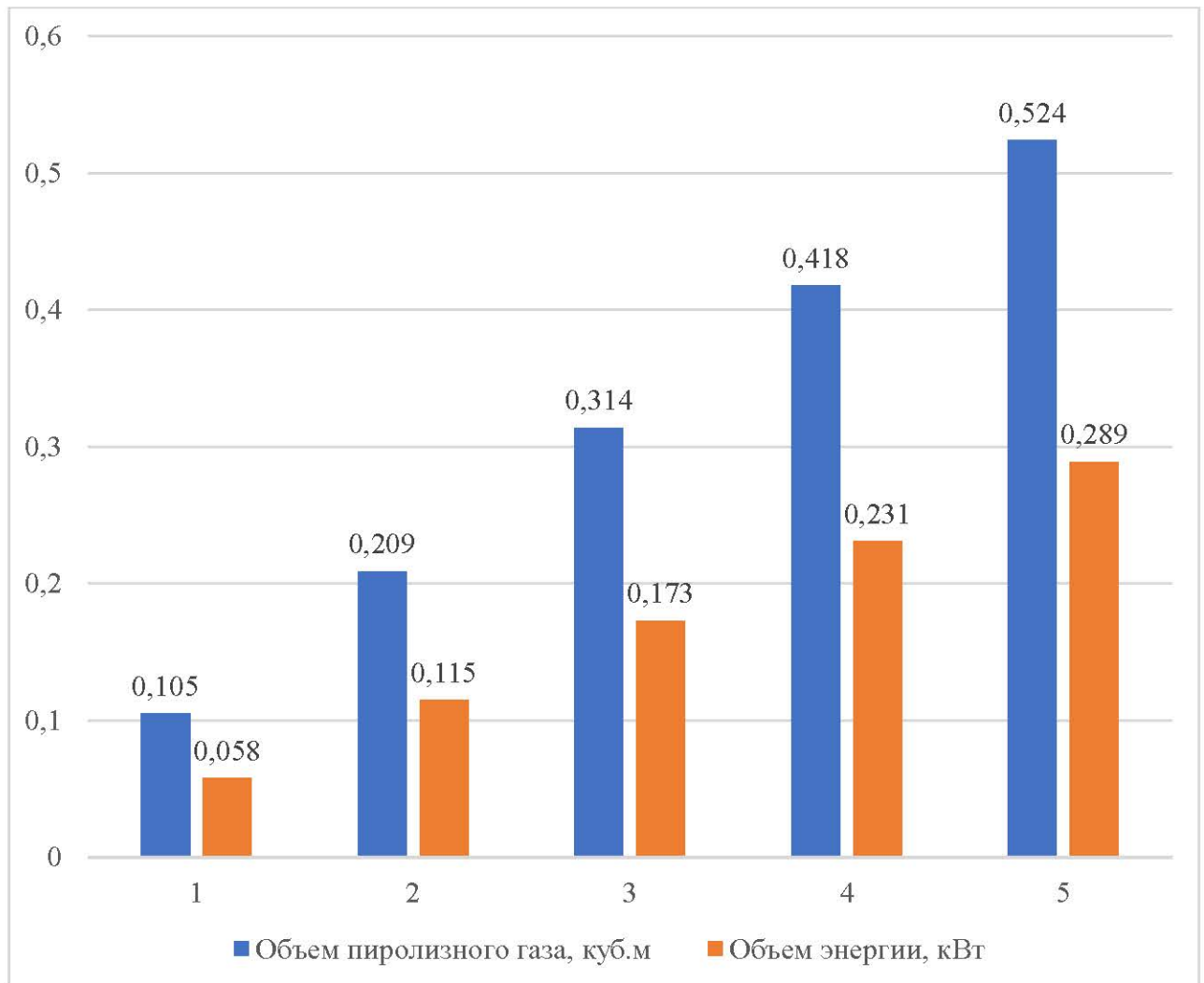
Рисунок 4.7 – График эквивалентных количеств энергий по соотношению к объемам пиролизного газа
