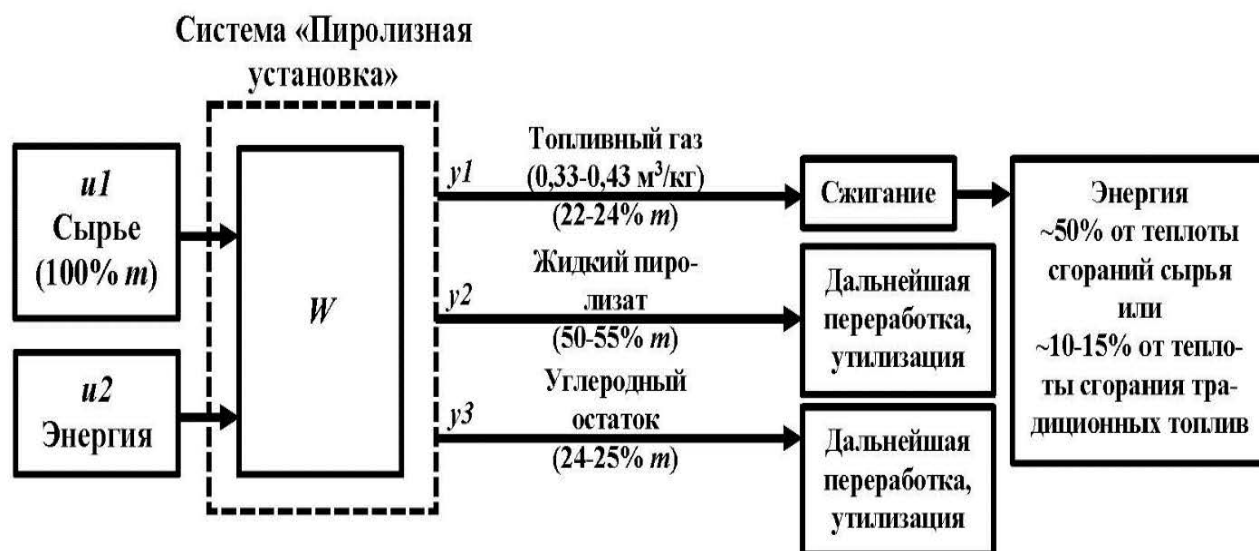
Рисунок 2.7 – Схема системы «Пиролизная установка» и ее материально-энергетического баланса
