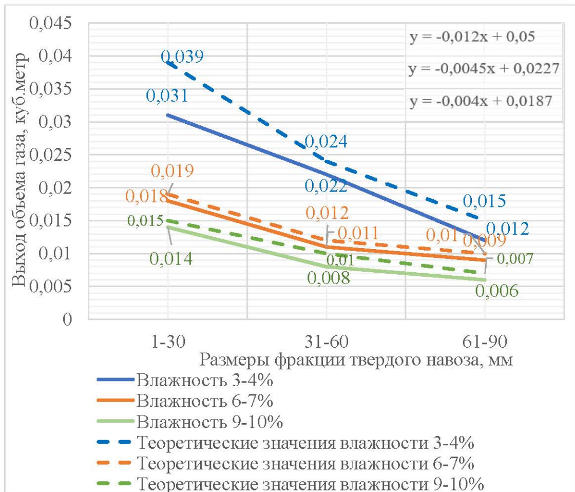
Рисунок 4.9 – Теоретические и экспериментальные значения выхода пиролизного газа
