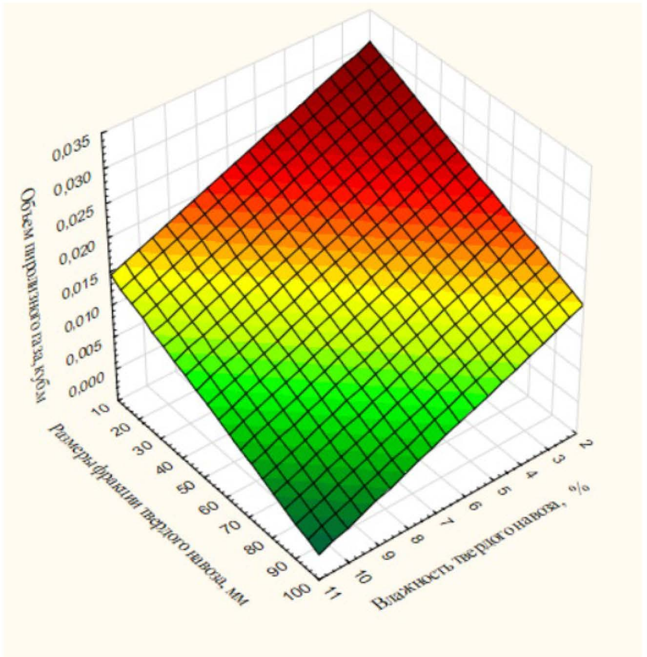
Рисунок 4.10 - Количество пиролизного газа, получаемое в зависимости от факторов влажности и размеров фракции твердого навоза
