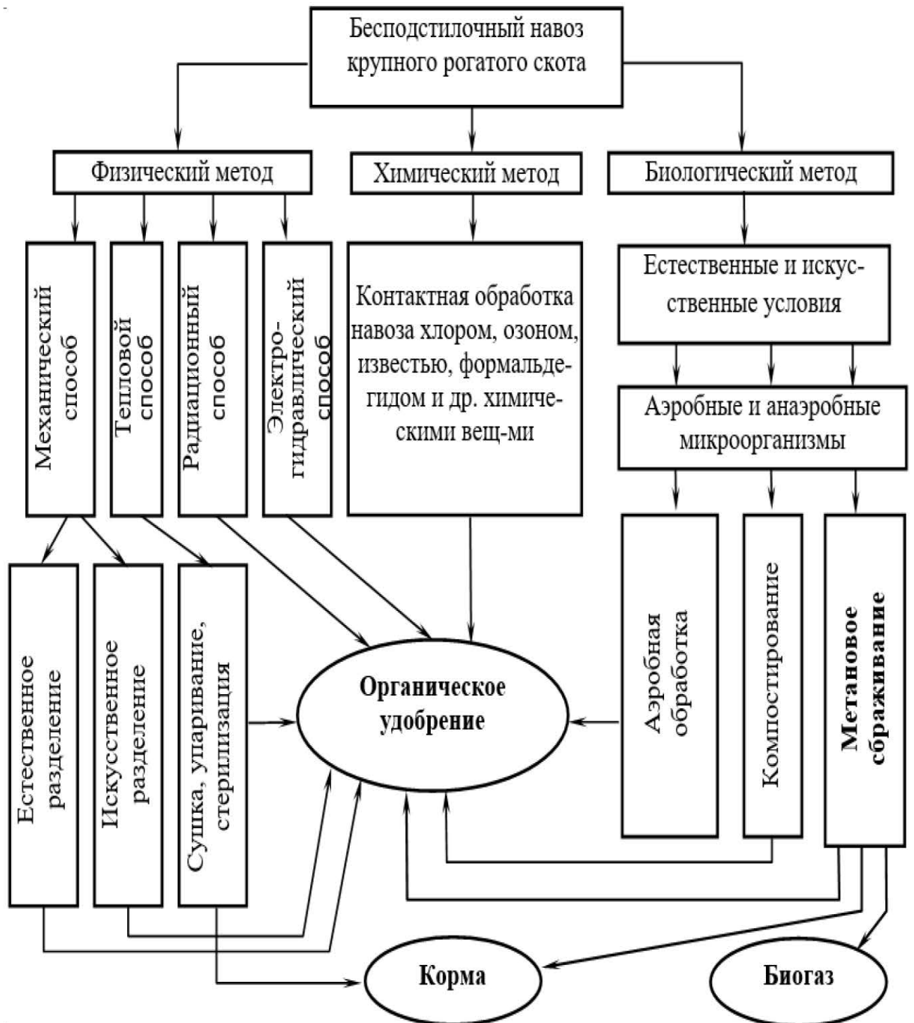
Рисунок 1.6 - Методы и способы переработки бесподстилочного навоза крупнорогатого скота [66]
