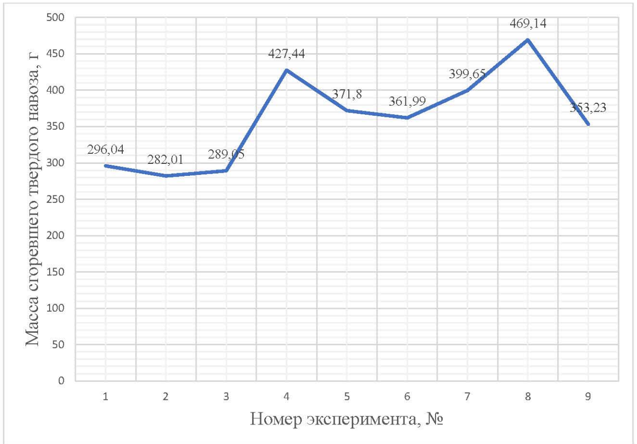
Рисунок 4.8 – График, описывающий массу сгоревшего твердого бесподстилочного навоза в термореакторе установки ГВА-1
