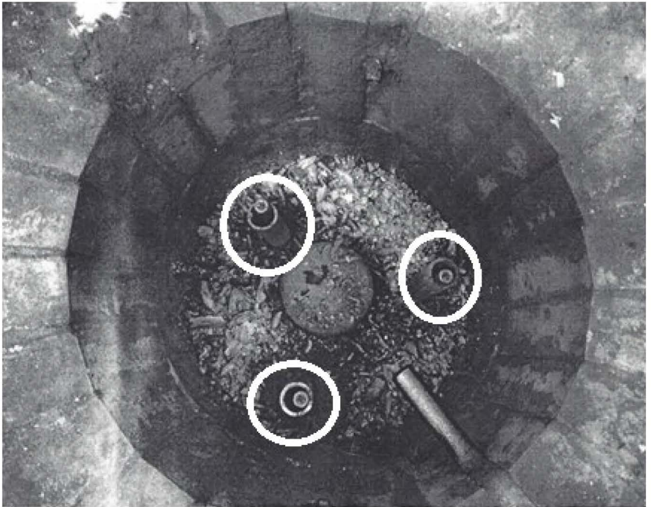
Рисунок 4.2 – Общий вид ТЭНов с кожухами
