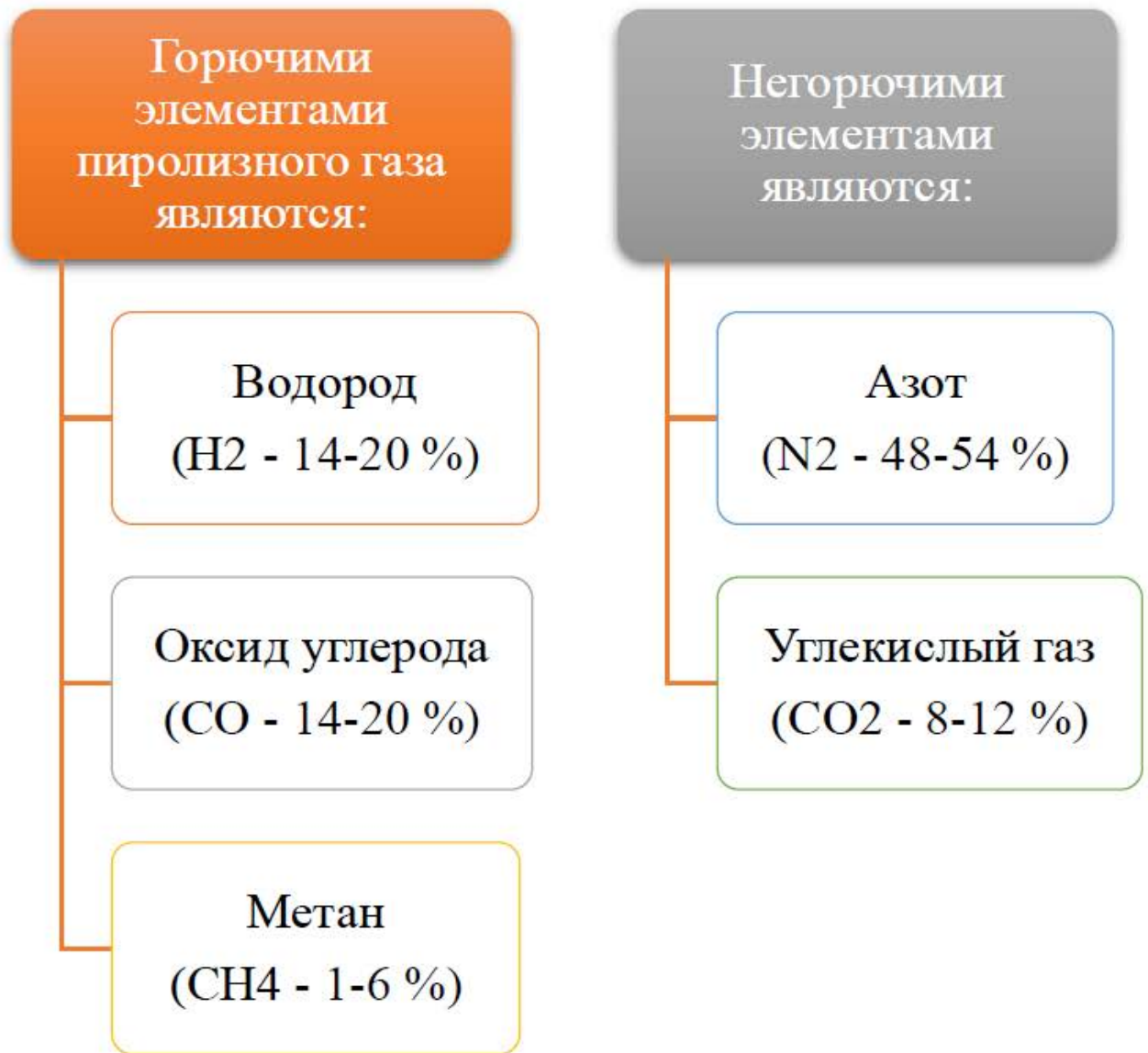
Рисунок 2.4 – Схема элементов пиролизного газа [6]
