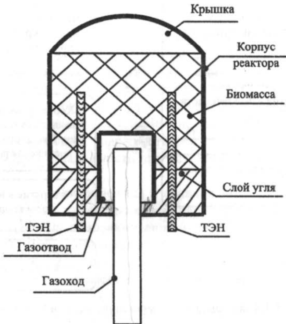
Рисунок 3.4 – Общий вид термореактора пиролизной установки ГВА-1
