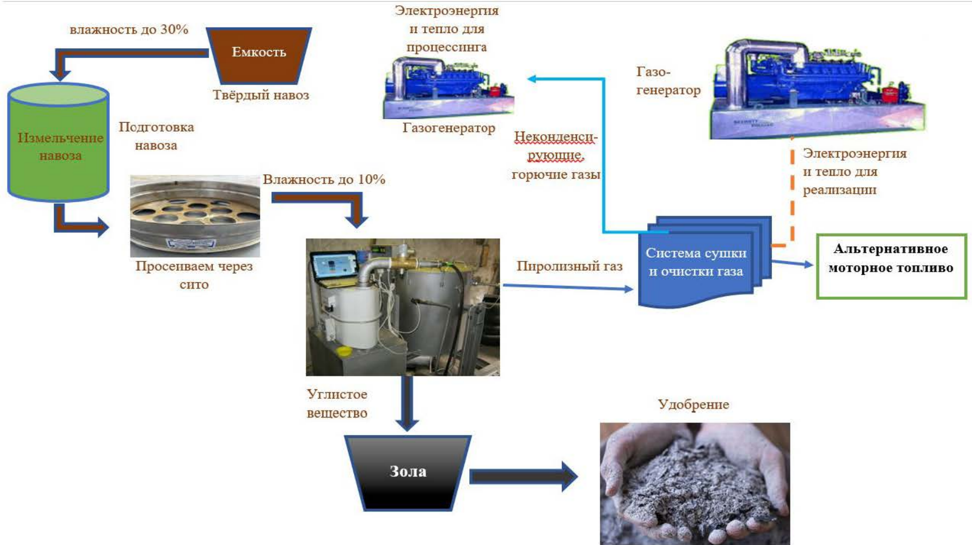
Рисунок 5.1 - Технологическая схема предлагаемой пиролизной технологии утилизации твердого бесподстилочного навоза
