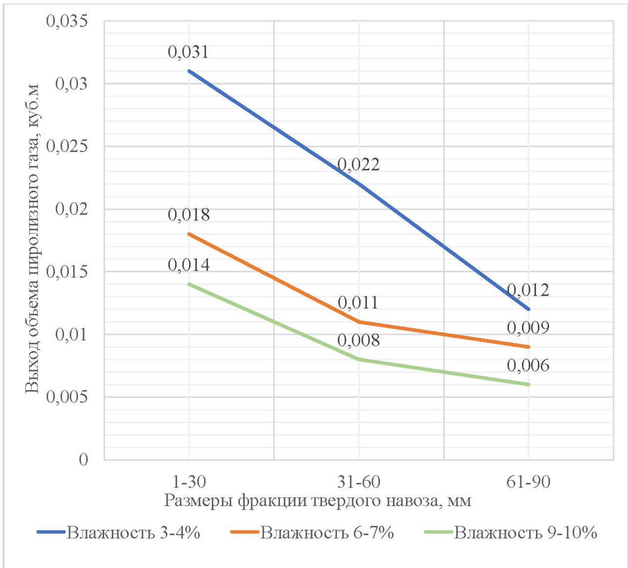
Рисунок 4.5 - Выход пиролизного газа в зависимости от параметров влажности и размеров фракций твердого бесподстилочного навоза
