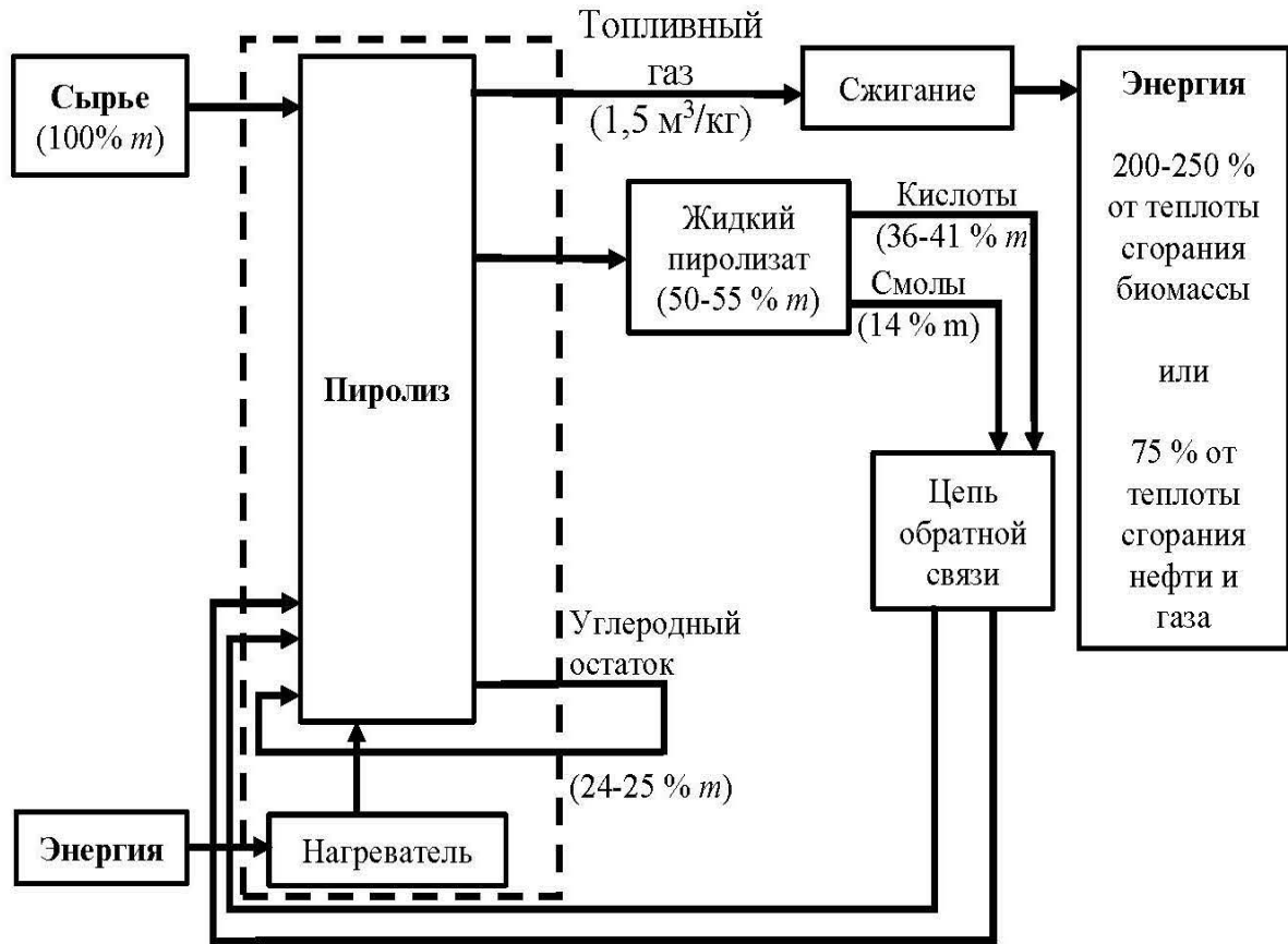
Рисунок 2.9 - Схема пиролиза в установке ГВА-1
