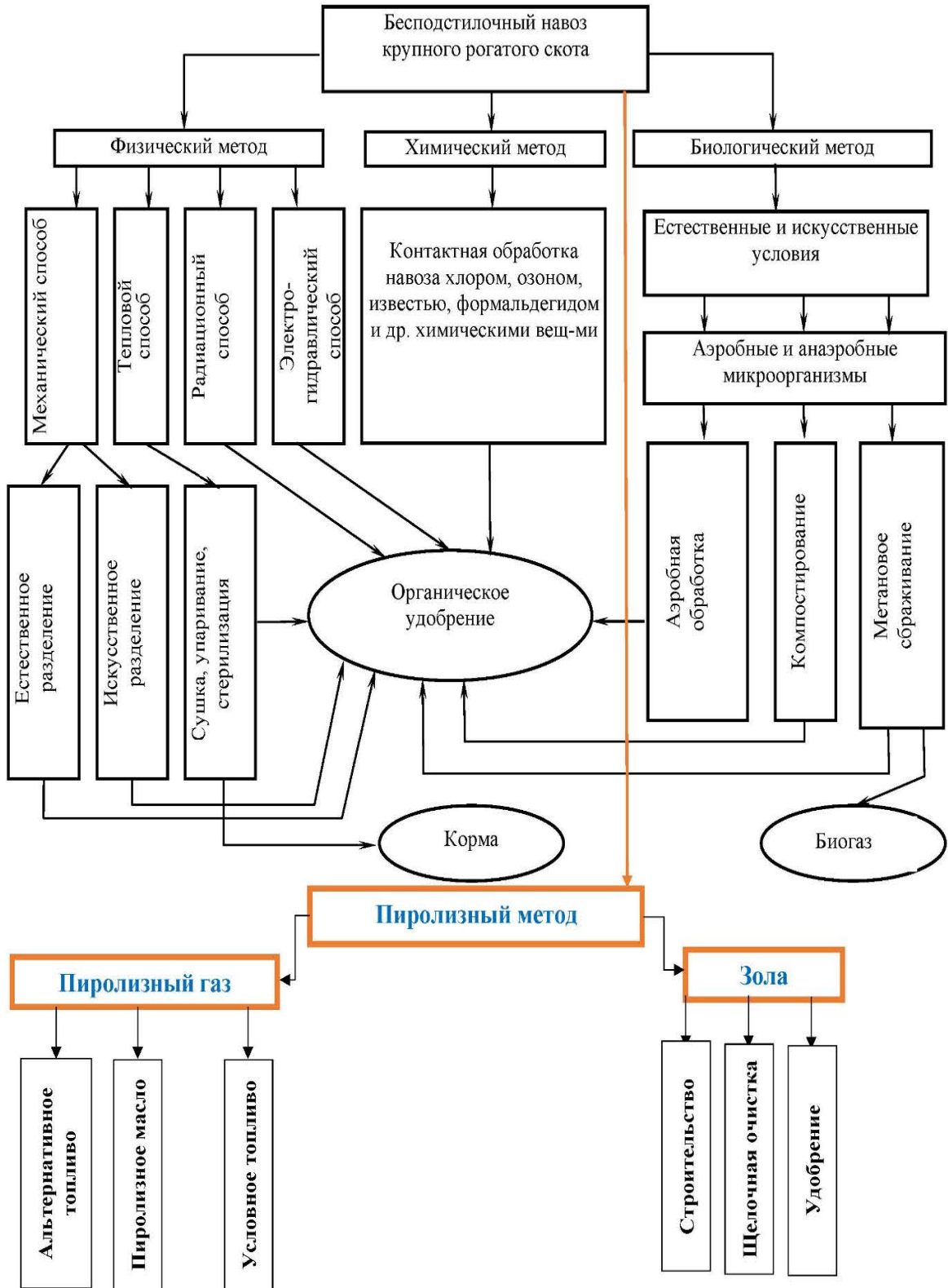
Рисунок 2.6 - Предлагаемая модернизированная схема по способам и методам утилизации навоза КРС - жидкого и твердого
