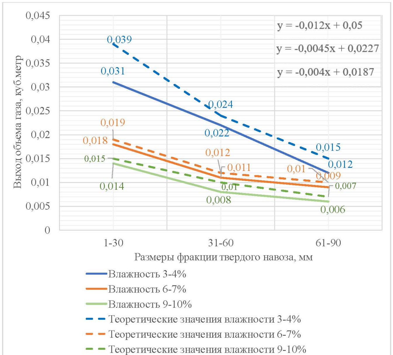
Рисунок 4.6 – Теоретические и экспериментальные значения выхода пиролизного газа
