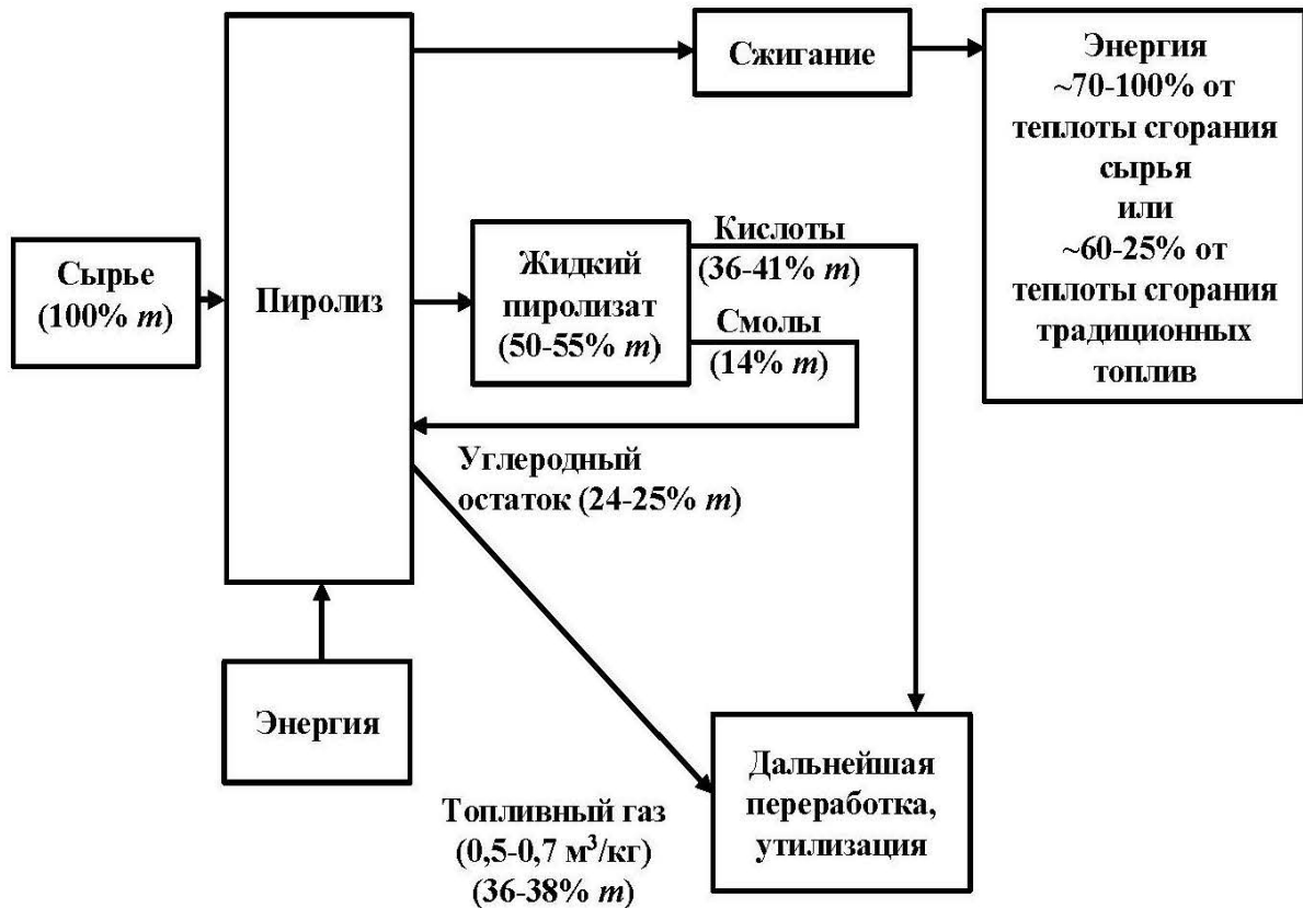
Рисунок 2.8 – Схема материально-энергетического баланса разработанного процесса пиролиза
