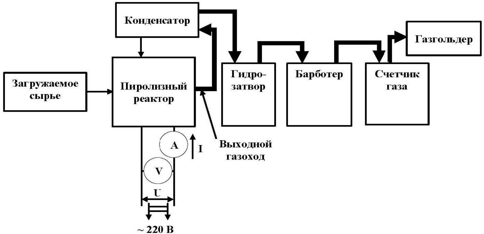
Рисунок 2.5 – Принципиальная схема пиролизной технологии Глушкова
