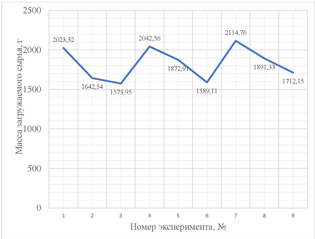
Рисунок 4.4 - График, описывающий массы измельченного навоза, забранных в тару объемом 14 л, г (при экспериментах)
