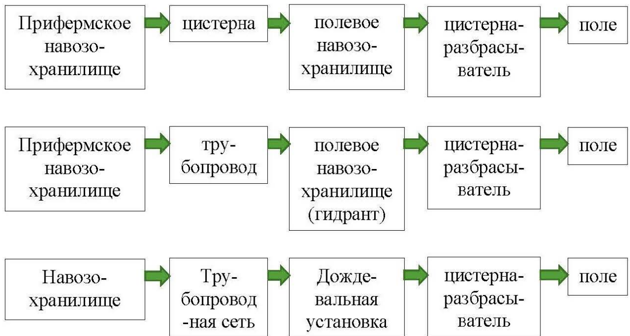
Рисунок 1.5 - Схемы по использованию бесподстилочного навоза
