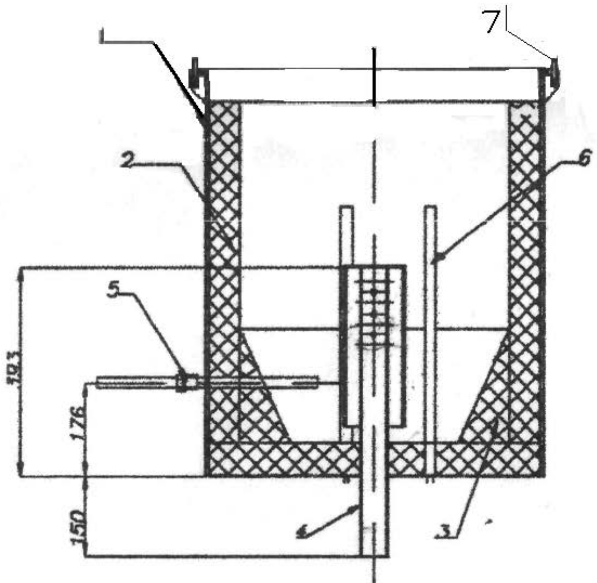
Рисунок 3.5 - Реакционная камера в сборе:
