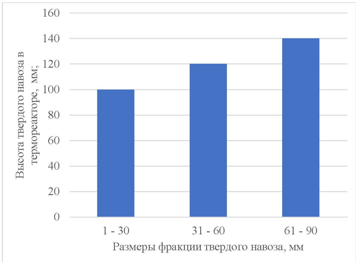
Рисунок 4.3 – Диаграмма по значениям заполнения реактора пиролизной установки в зависимости от размеров фракций измельченного навоза
